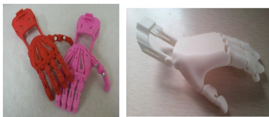
Figura 10. Ejemplo de prótesis de mano elaboradas con impresoras 3D [15]
