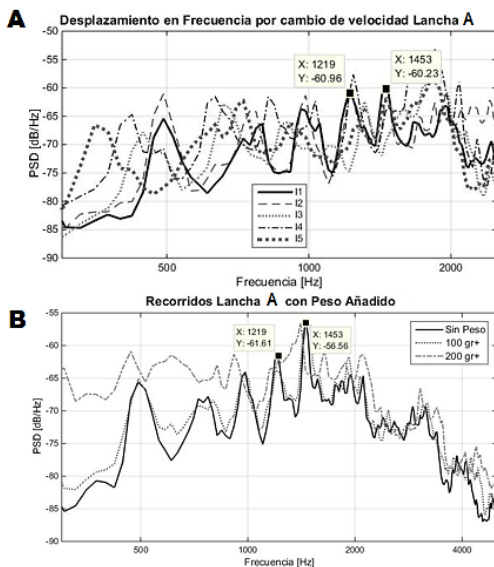
Figura 30. Invariancia en algunas frecuencias con el cambio de velocidad y peso
