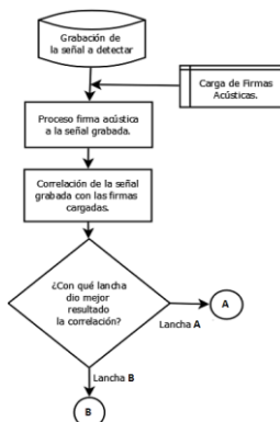
Figura 27. Comparación entre la señal capturada y las firmas acústicas previamente almacenadas
