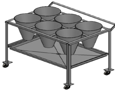
Figura 1. Prototipo drenadora de sangre
