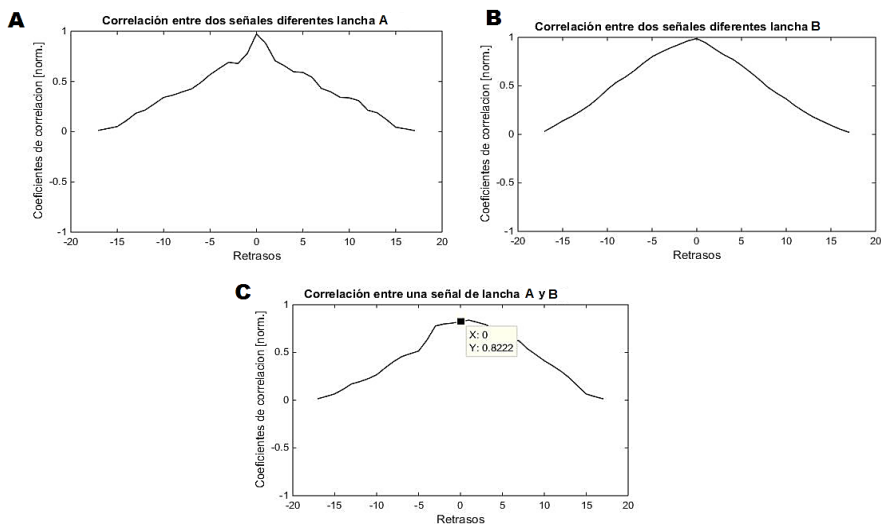
Figura 32. Representación del resultado de correlación entre A) dos señales de lancha A, B) dos señales de lancha B y C) entre una señal de A y B
