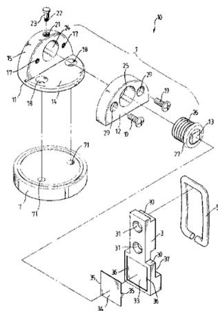
Figura 6. Unidad de soporte fija imantada desarrollada [6]
