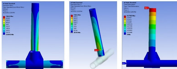
Figura 9. Resultados de las pruebas mínimo y máximo esfuerzo, mínima y máxima deformación
