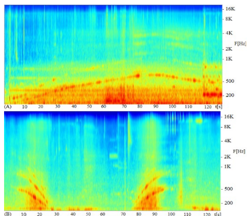
Figura 11. (A) Audio estéreo de un vehículo del metro en circulación. (B) De un vehículo del metro arribando y saliendo en una estación. Azul oscuro: nivel de presión sonora entre -10 a 10 dB, azul aguamarina: entre 15 a 35 dB, amarillo: entre 35 a 60 dB, rojo: entre 60 a 80 dB
