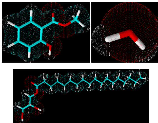
Figura 6. Estructuras optimizadas representadas en 3D de los sustratos usados por la enzima Lipasa para la catálisis hidrolítica: a) salicilato de metilo, b) agua, c) monoestearato de glicerilo
