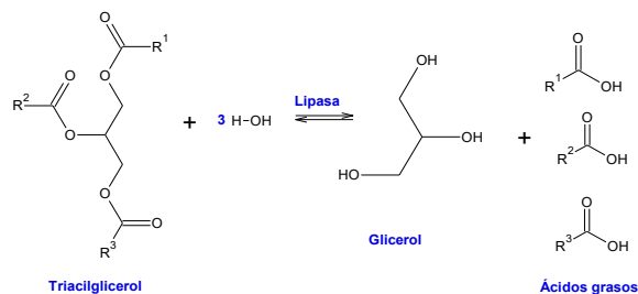
Figura 1. Hidrólisis de ácidos grasos por la enzima lipasa
