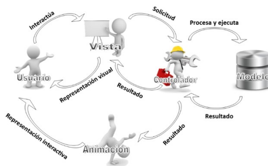
Figura 5. Modelo MVAC
