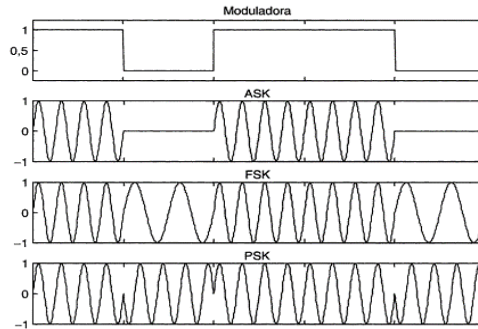
Figura 3. Modulaciones radio digitales
