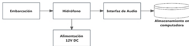
Figura 25. Diagrama de flujo para la obtención de datos
