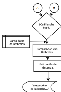
Figura 28. Diagrama de flujo para el porcentaje de detección y la distancia aproximada
