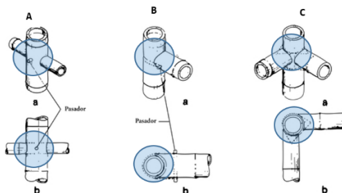
Figura 8. Amarres para estructuras de bambú a base de cinta de PET reciclado
