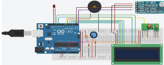
Figura 14. Diseño del receptor del sistema de cronometraje
