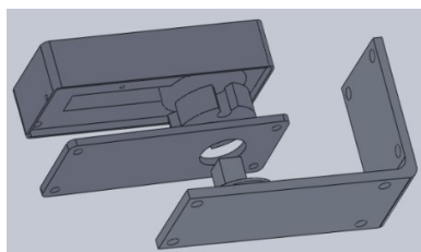
Figura 12. Sistema interno dentado en cuadrante
