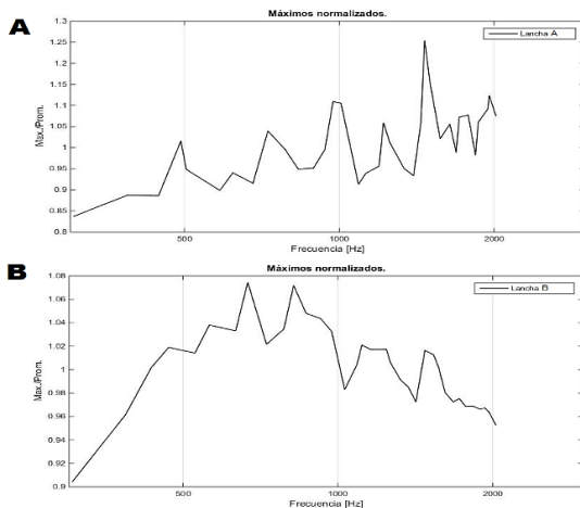
Figura 31. Representación de firma acústica de ambas lanchas A y B
