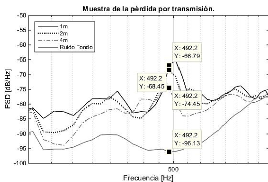
Figura 33. Pérdida por transmisión usada para estimar distancias al hidrófono
