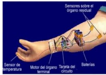
Figura 5. Prótesis Mioeléctrica [6]
