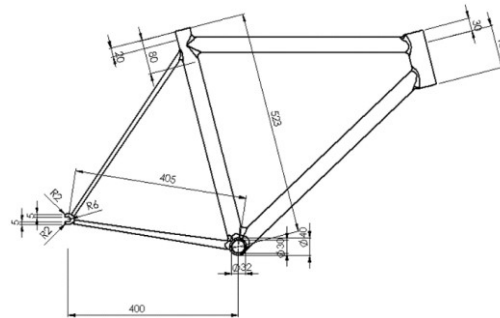
Figura 2. Vista frontal del marco 2D
