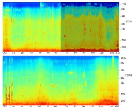
Figura 10. (A) Punto 2 con tráfico habitual, (B) punto 2 en el día sin carro. Azul oscuro: nivel de presión sonora, azul aguamarina: 15 a 35 dB, amarillo: entre 35 a 60 dB, y rojo: 60 a 80 dB
