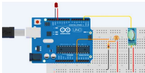
Figura 11. Diseño del módulo transmisor
