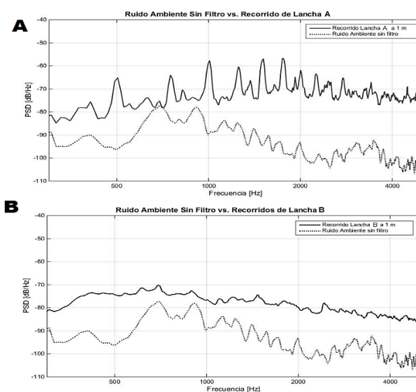
Figura 29. Comparaciones de los pasos de las lanchas A y B con respecto al ruido de fondo
