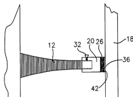
Figura 8. Sujetador tipo gancho y lazo planteado por Murphy
