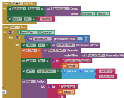
Figura 18. Diagrama de bloques del Aplicativo móvil
