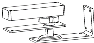
Figura 11. Perfil de bisagra en conjunto soporte inferior
