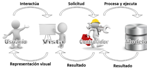
Figura 4. Modelo MVC
