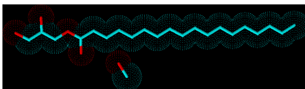
Figura 7. Estructuras 3D del \text{CH}_3\text{OH} y el monoestearato de glicerilo
