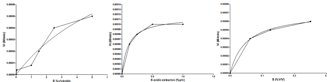
Figura 4. Gráficas de Michaelis y Menten de los sustratos: a) aceite de oliva extra virgen, b) monoestearato de glicerilo, c) salicilato de metilo
