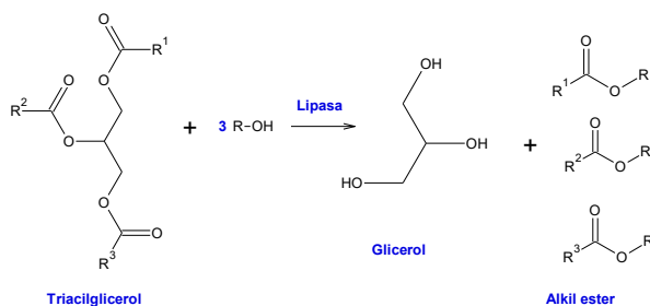
Figura 2. Reacción de transesterificación catalizada por la enzima Lipasa
