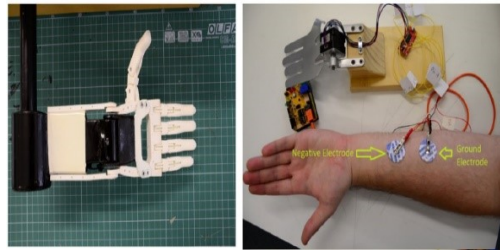
Figura 11. Modelo de prótesis impresa en 3D (izquierda) y toma de señales mioeléctricas para caracterización (derecha) [15]
