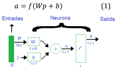
Figura. 2 Diagrama de una red neuronal [10]
