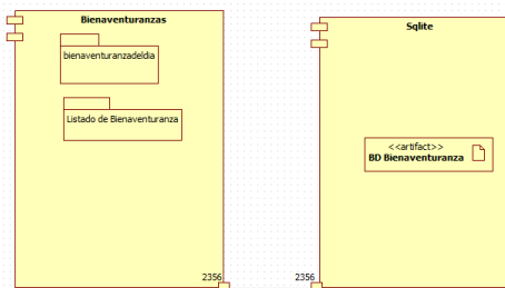
Figura 5. Diagrama Arquitectónico de la aplicación móvil de las bienaventuranzas
