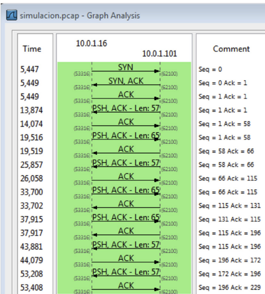
Figura 11. Diagrama de tiempos comunicación TCP.
