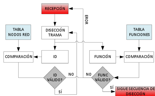
Figura 7. Diagrama de flujo recepción de trama protocolo red HAN.
